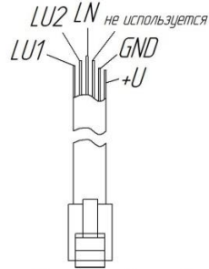
Рис. 3 Схема подключения устройства через телефонные кабели напрямую к блоку вызова и коммутатору (без использования розетки ТЖС-6С)
