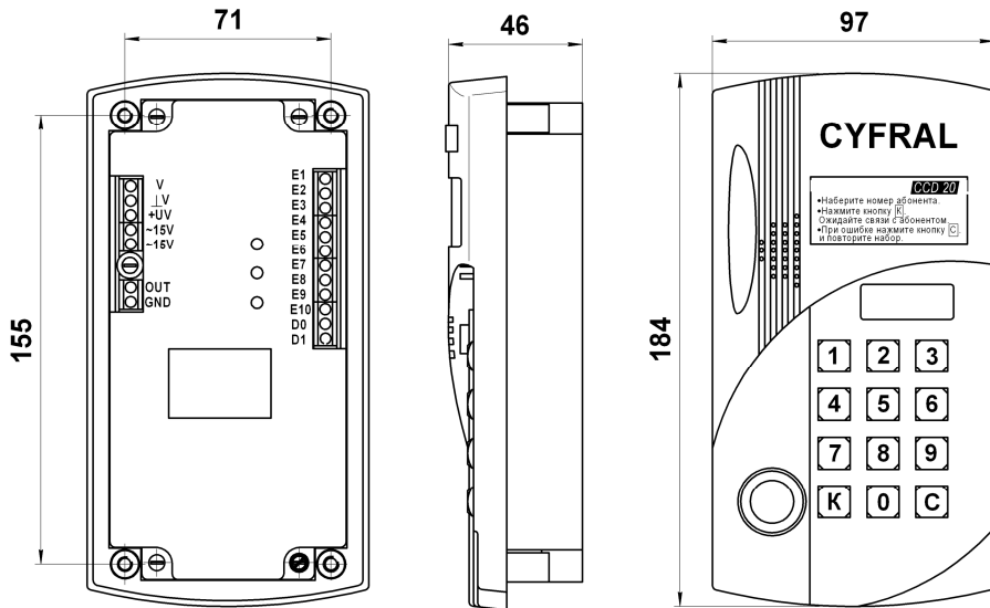
Рисунок А.1 Габаритные и установочные размеры блоков вызова ЦИФРАЛ ССD-20/ТС, ЦИФРАЛ ССD-20/ТСV, ЦИФРАЛ ССD-20/Р, ЦИФРАЛ ССD-20/РV
